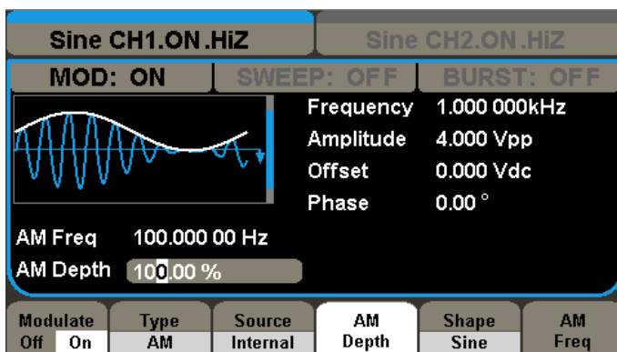
Рисунок 1-15 Вид интерфейса для режима модуляции
