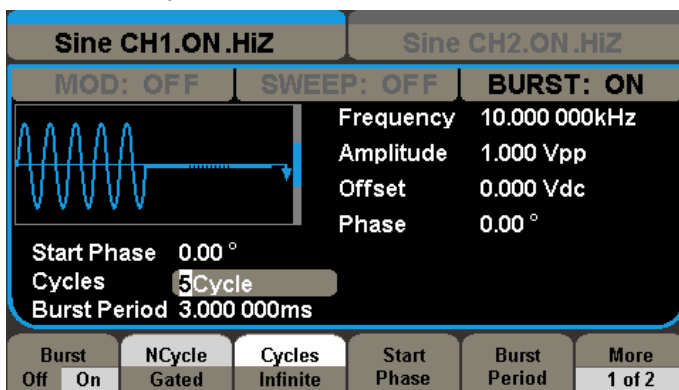
Рисунок 3-8 Пример получения сигнала пачки
