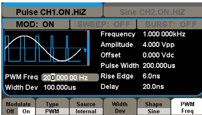
Рисунок 2-40 Вид интерфейса широтно-импульсной модуляции (PWM)
