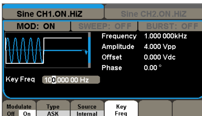
Рисунок 2-34 Вид интерфейса амплитудной манипуляции (ASK)
